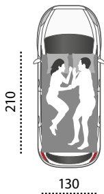
SMALL Art. MCF/01 Maggiolina Carbon Fiber Small, Schalen aus Kohlenstofffaser. Für 2 Erwachsene geeignet.
